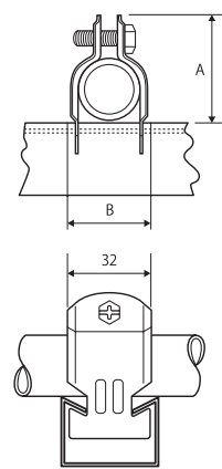
HL レベル金具用片サドル
