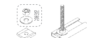
Dバー 取付例
